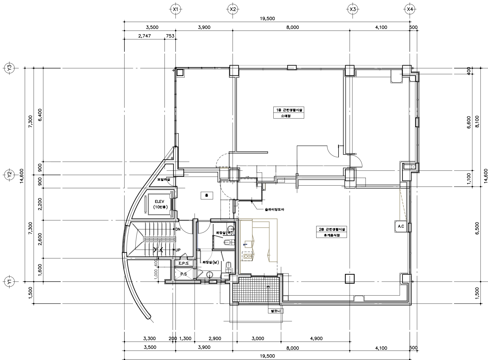
2층 평 면 도 (설계변경후) 축척 : 1/ 100
