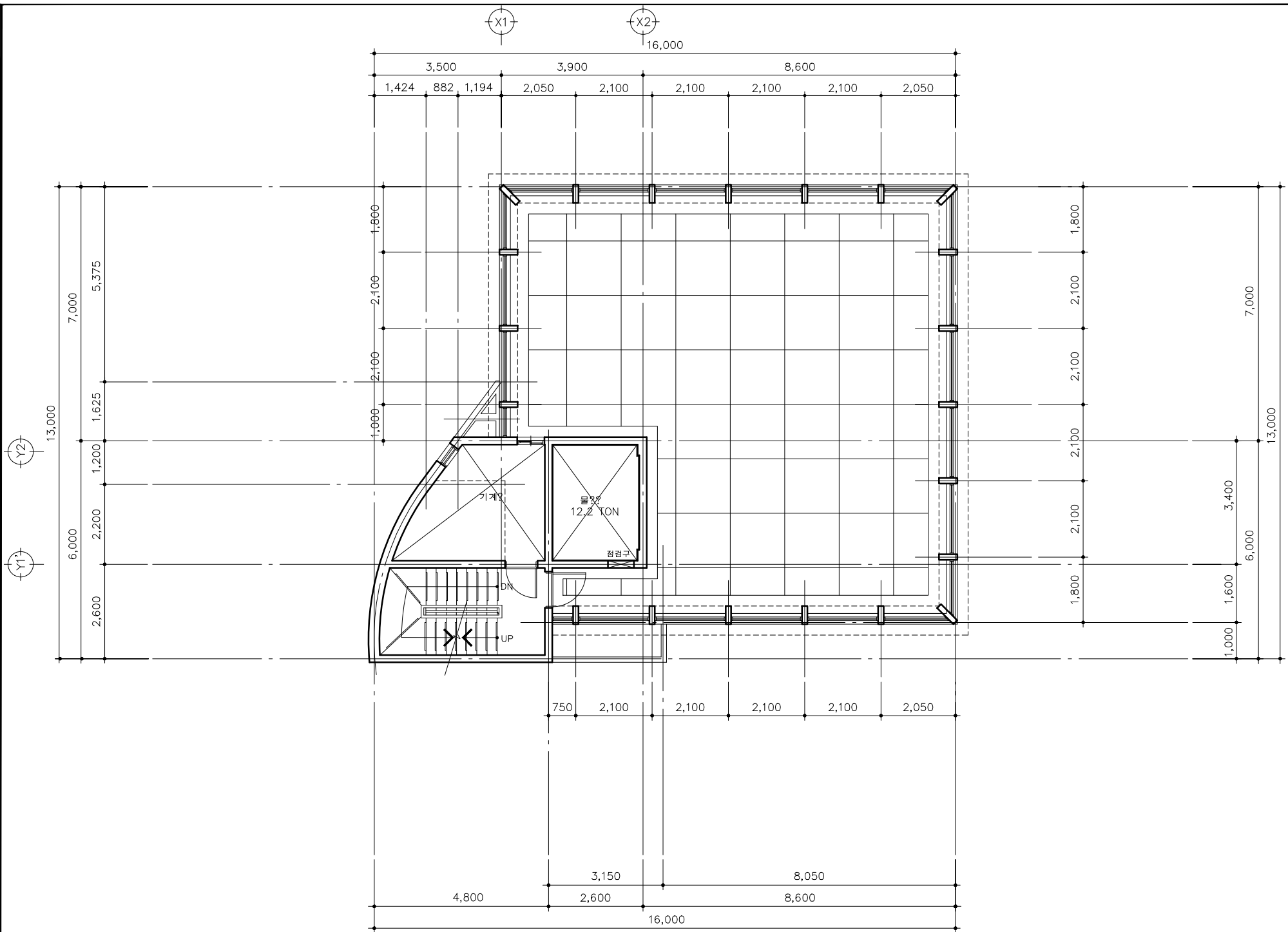
옥탑1층 평면도
