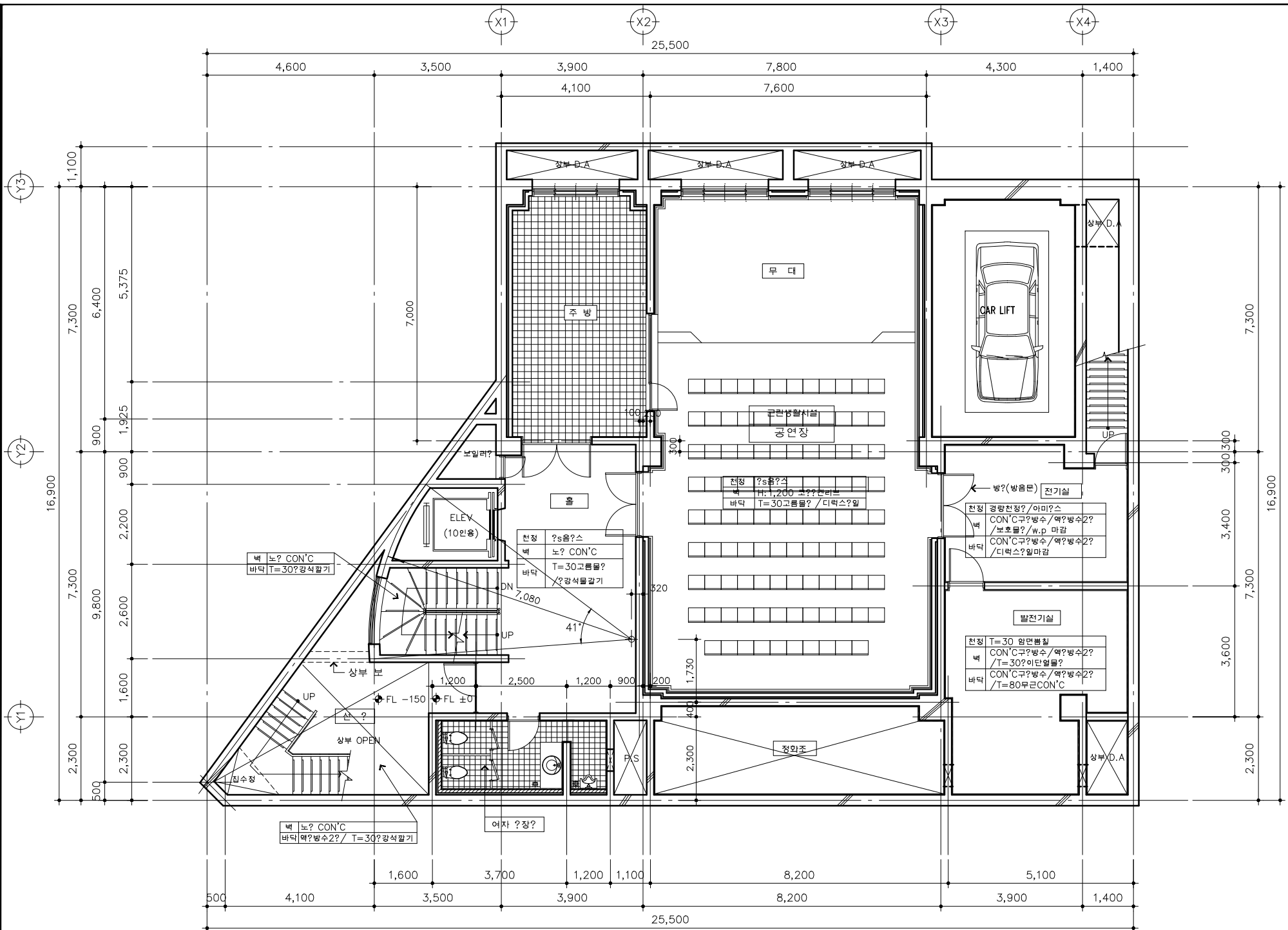
지하 1층 평면도
